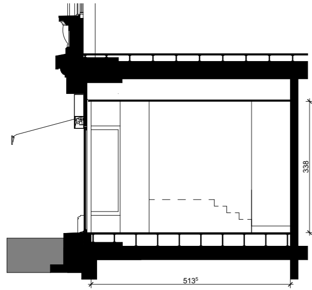
COUPE A
