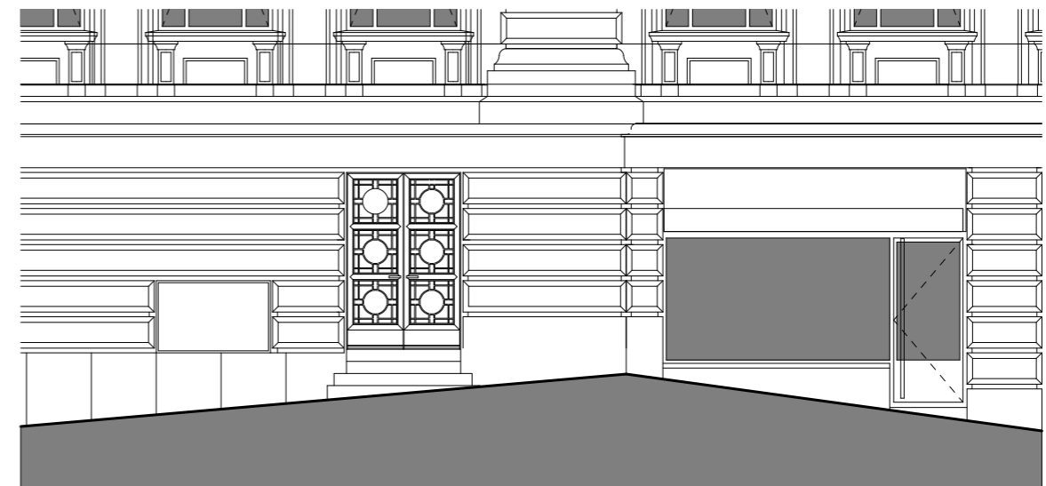
ELEVATION OUEST
